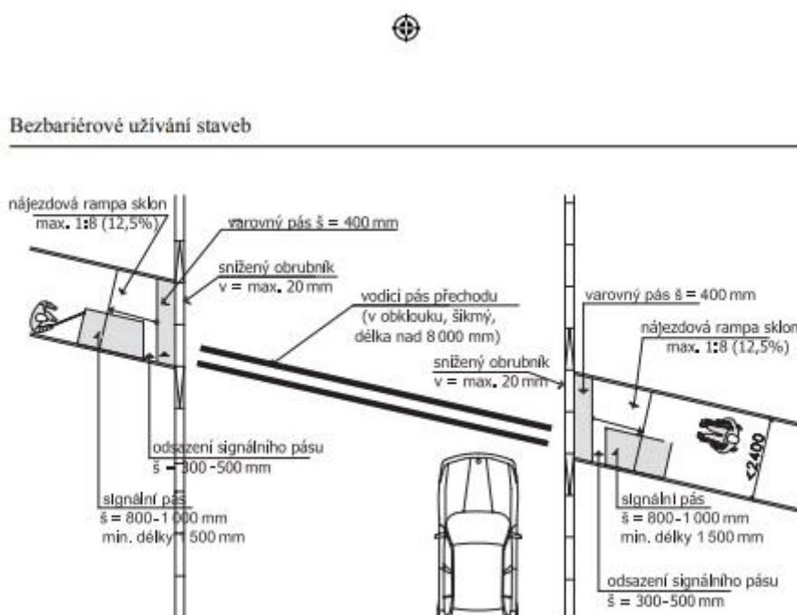
Obr. 110 Místo pro přecházení vedené šikmo, chodník šířky menší než 2400 mm
